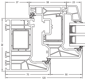
Schüco LivIng 82 AD
