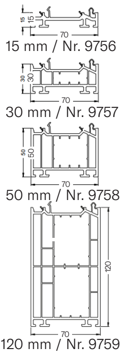
Schüco CT70
