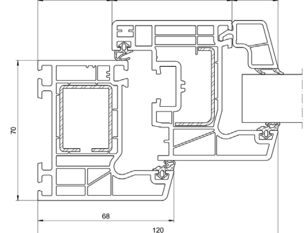
Schüco CT70
