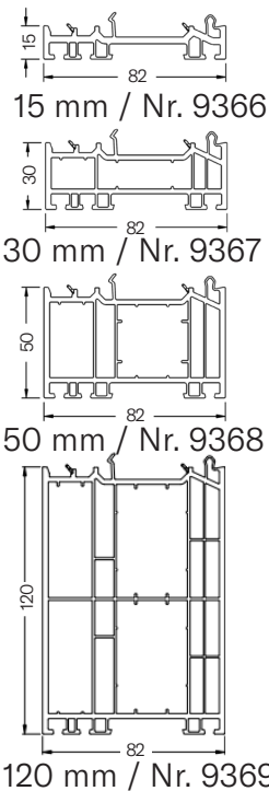
Schüco LivIng 82
