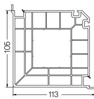
Eckkopplung 90° Nr. 9811s
