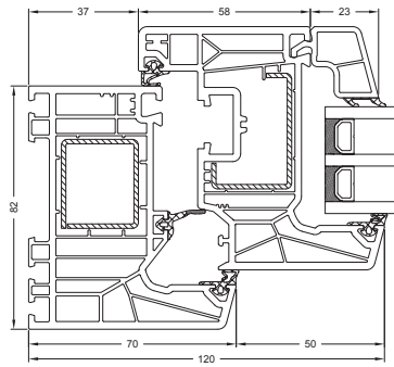
Schüco LivIng 82 MD
