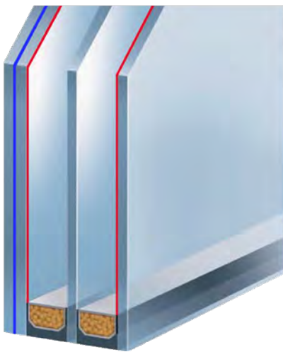
Aufbau einer einbruchhemmenden Verglasung mit P4A (hier als 3-fach Glas)
